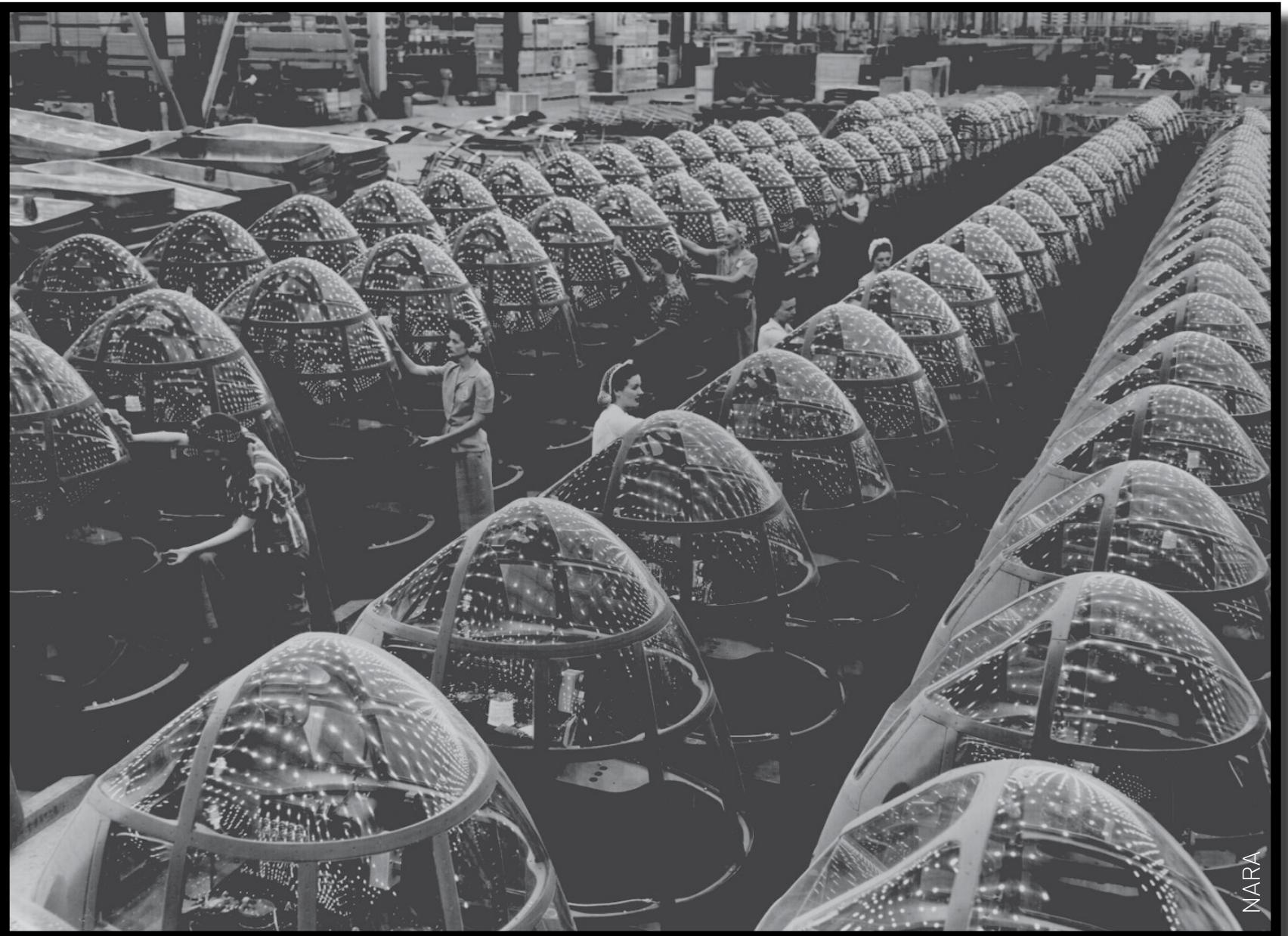
Usine de Douglas Aircraft à Long Beach en Californie, nez de bombardiers d'attaques A-20 en train d'être assemblés par des ouvrières en octobre 1942
