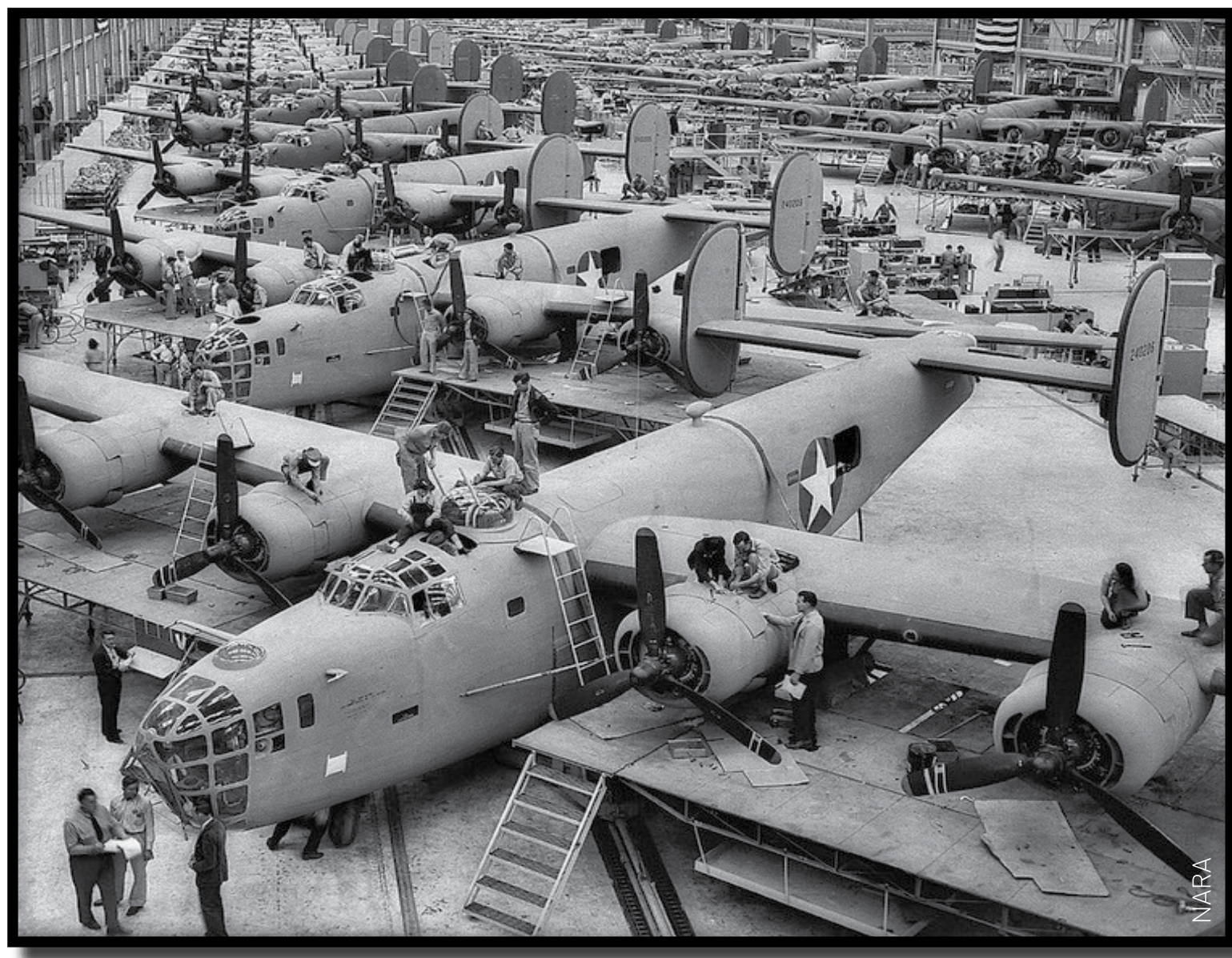
Ligne de production des B-24 dans l'usine Consolidated de Dallas Fort Worth
